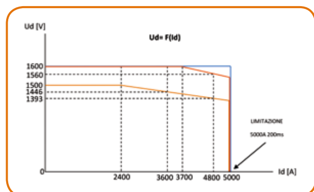
Caratteristica di regolazione, tensione nominale di rete 660Vac (rossa) - 660Vac +10% (blu) - 660Vac - 10% (arancio)
